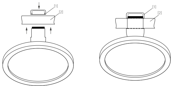
Рис. 2. Установка светильника
