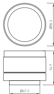
Рис. 1. Чертеж и габаритные размеры
