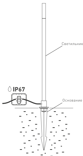
Рис. 2. Установка и подключение светильника
