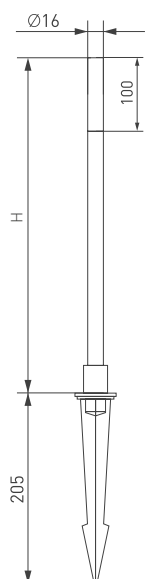
Рис. 1. Чертеж и габаритные размеры
